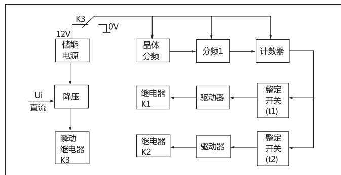
图1 继电器原理框图
