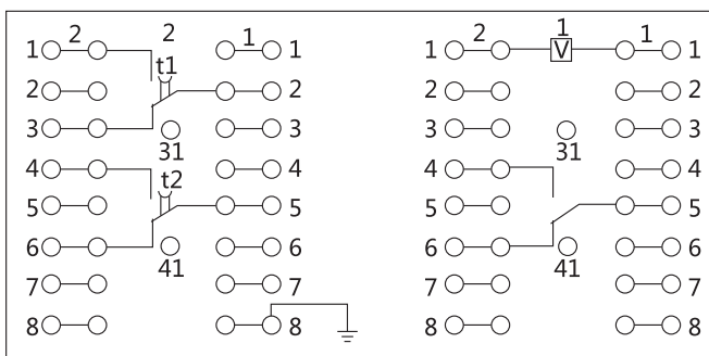
图2 面板示意图
