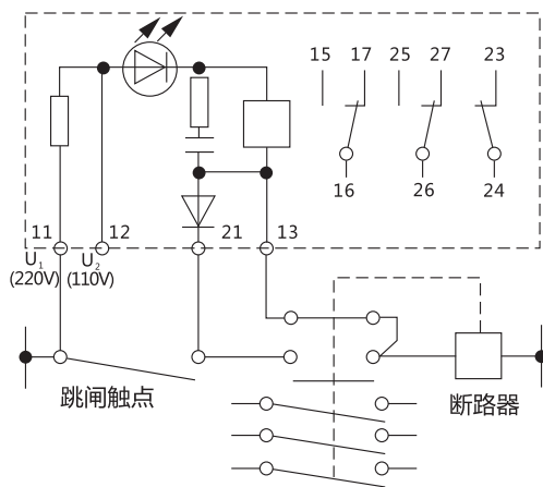
跳闸回路监视
