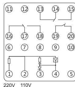
DJS-4 内部接线图 (正视)
