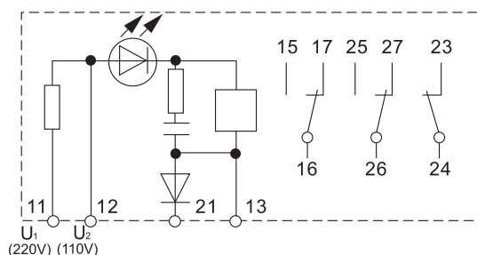
图 2 DJS-1 内部接线图 (背视)
